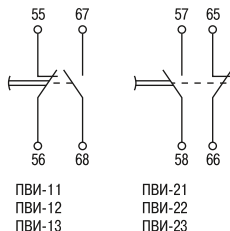
Рисунок 7 Электрические схемы ПВИ
