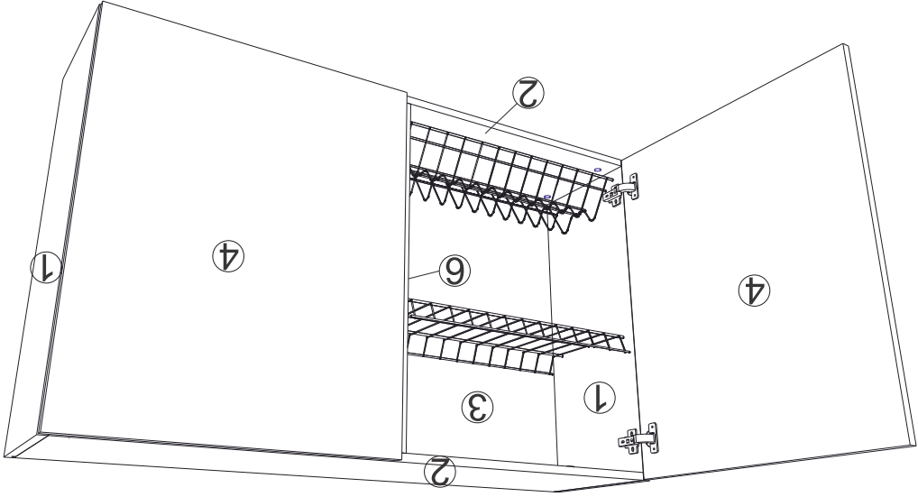
Схема сборки изделия
