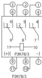
Рисунок 2. Схемы подключения
