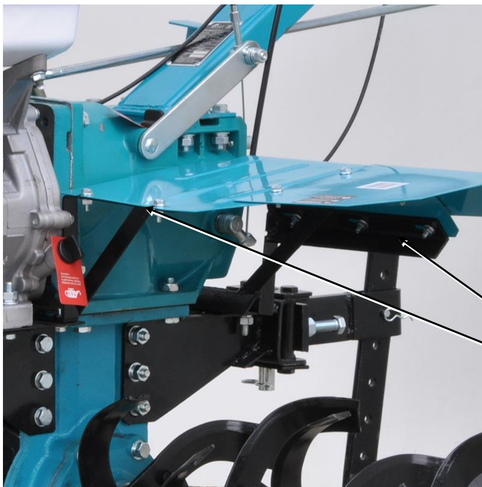
Панки крепления щитков
