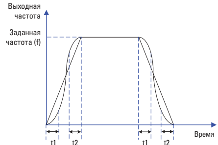
Кривая А: схема S-кривой ускорения/торможения А
