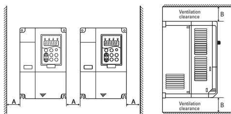
Монтажная схема верхнего единичного устройства
