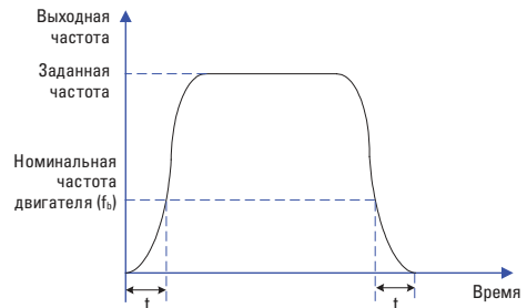
Кривая В: схема S-кривой ускорения/торможения В
