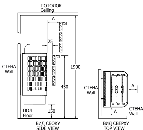
Рис. 1 | Минимальные безопасные расстояния (мм) Fig. 1 | Minimum safety distances (mm)
