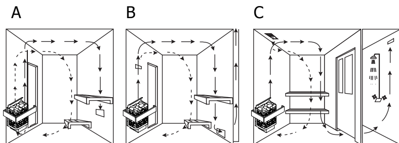
Рис. 6 | Вентиляция Fig. 6 | Air Ventilation
