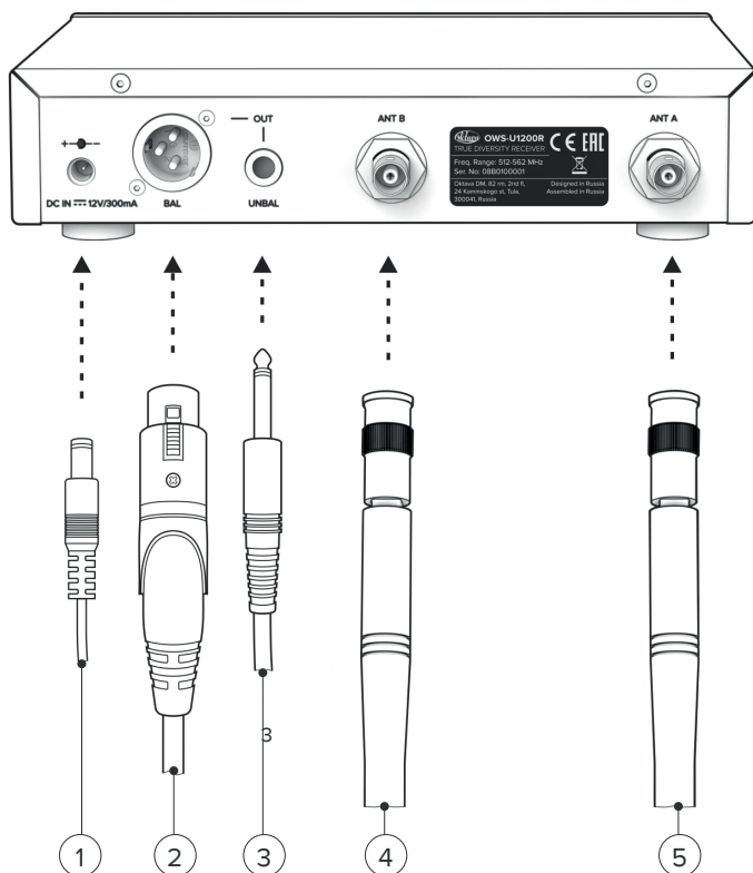
Схема 1. (1. Питание, 2. XLR, 3. Jack , 4-5. Антенны.)
