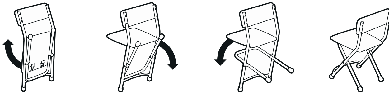
(рис. 5) Схема раскладывания стула с мягкой обивкой
