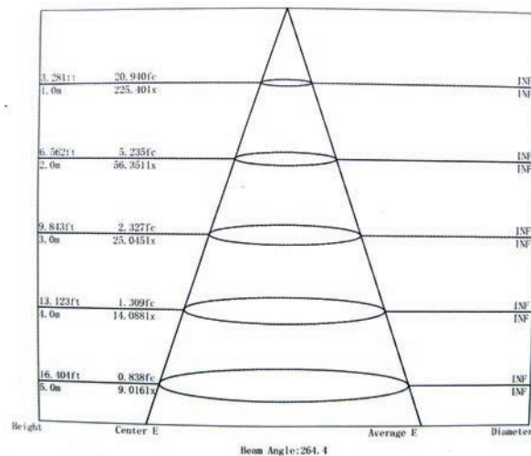
Кривая распределения света
