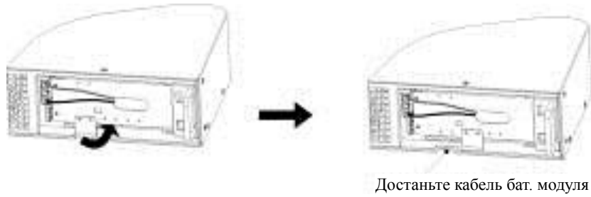
Рисунок 9 Удаление сепаратора кабеля ИБП
