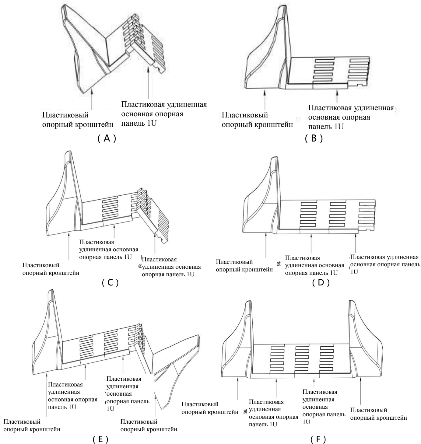
Рисунок 12: Установка увеличенной основной опоры EBP
