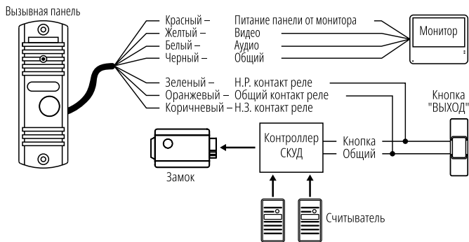
Схема подключения вызывной панели LEGEND к контроллеру СКУД
