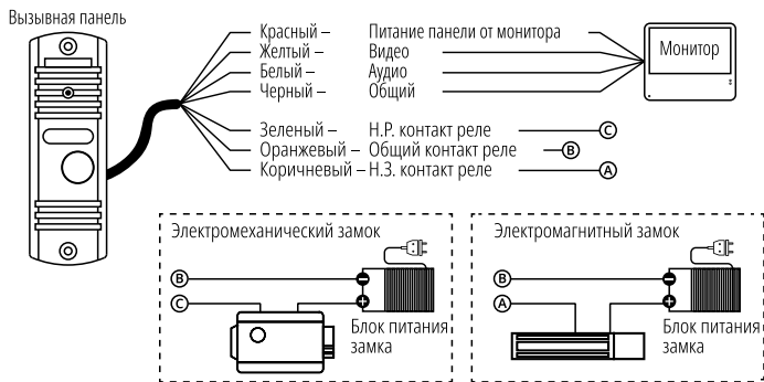
Схема подключения вызывной панели LEGEND
