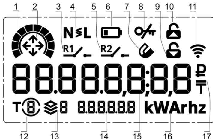
Рисунок 2. Отображаемые символы и знаки на ЖКИ
