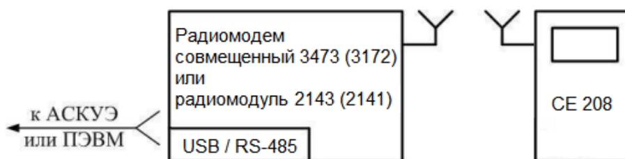
Рисунок 11. Схема подключения счетчика через радиointерфейс
