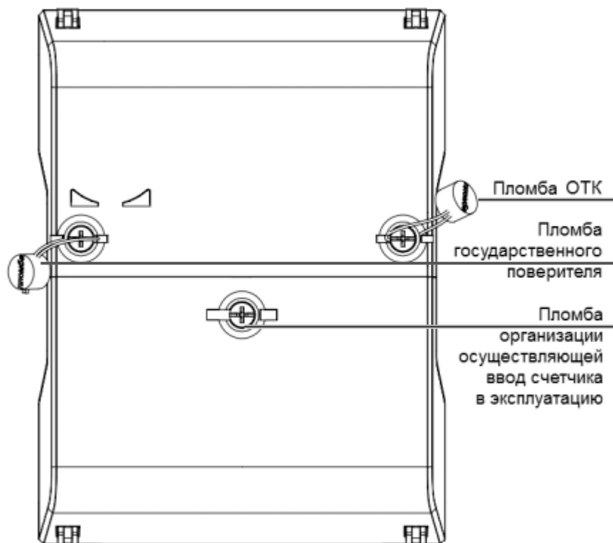
Рисунок 71. Пломбирование счетчика в корпусе S8
