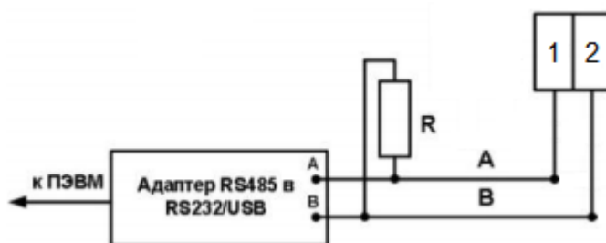
Рисунок 13. Схема подключения интерфейса RS-485 счетчика
