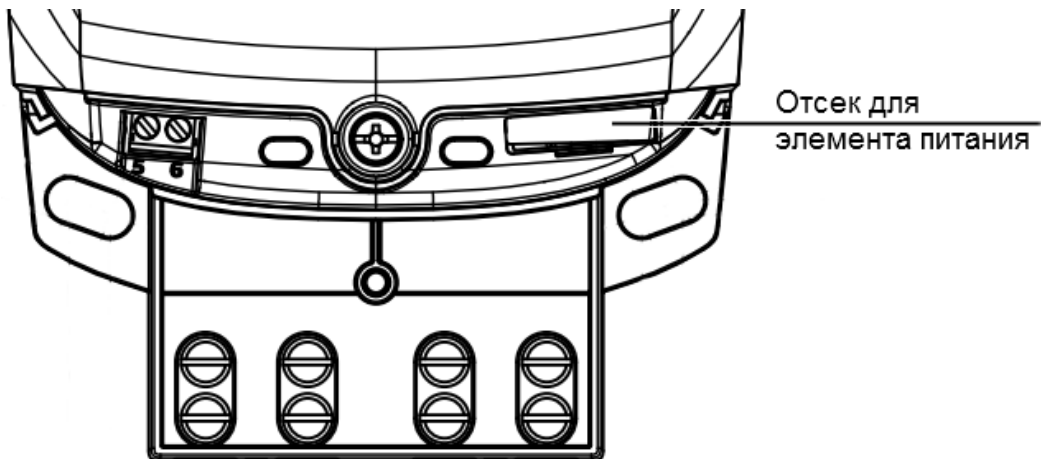
Рисунок 72. Отсек для элемента питания счетчика в корпусе S51, S53
