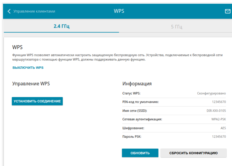
Рисунок 90. Страница для настройки функции WPS.
