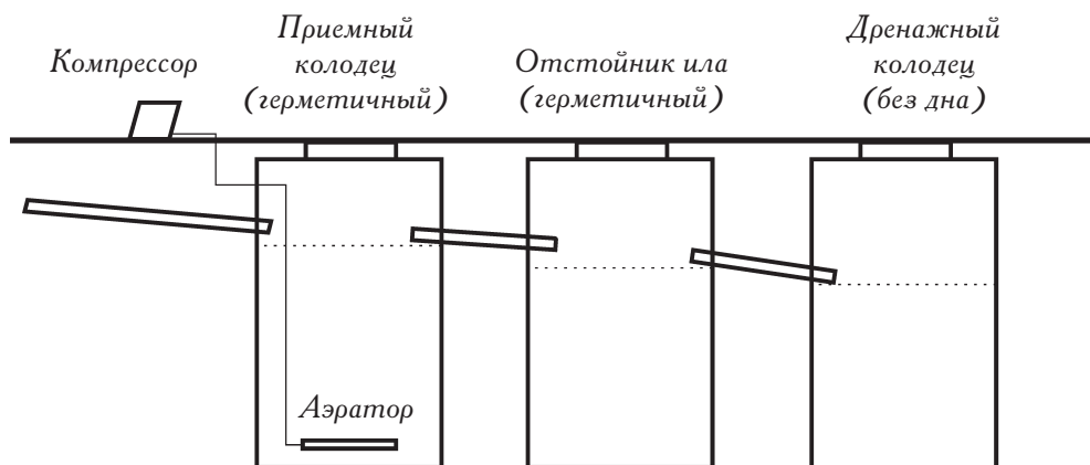
Рис. 2. Схема устройства трехкамерного септика с аэрацией
