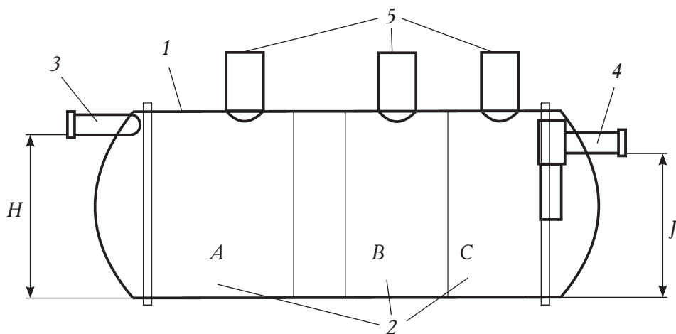
Рис. 1. Трехкамерный септик. Схематичное изображение. 1 — корпус септической части водоочистного сооружения, 2 — внутренние секции (А, В, С), разделенные блокираторами (гидрозатворами), 3 — патрубок подачи исходной канализационной сточной воды, 4 — отвод очищенной воды, 5 — вентиляционные люки для дозагрузки биопрепаратов и чистки
