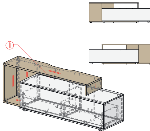
УНИВЕРСАЛЬНОЕ W3 / DI 171T005 1745 X 450 X 566
