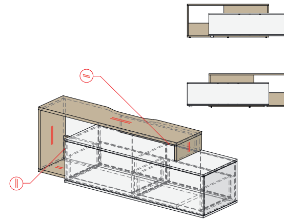
УНИВЕРСАЛЬНОЕ W3 / DI 171T006 1745 X 450 X 566
