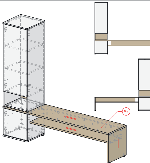
УНИВЕРСАЛЬНОЕ W3 / DI 171T002 1770 X 400 X 1632
