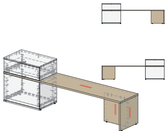
УНИВЕРСАЛЬНОЕ W3 / DI 171T001 1980 X 400 X 642
