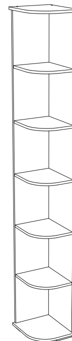
ЛШ-10 (Угловой стеллаж) 2212x300x348 (ВxШxГ)
