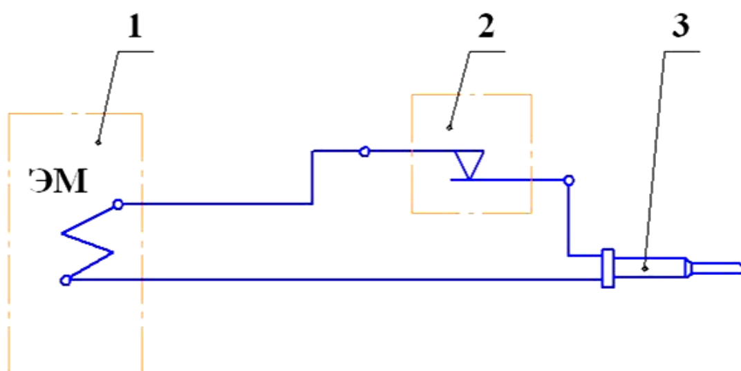
Рис.3 Схема электрическая.
