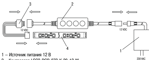
Рисунок 8 – Схема параллельного подключения многоцветной светодиодной RGB-ленты к блоку питания и контроллеру
