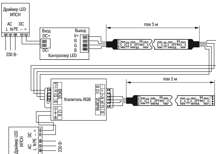
Рисунок 10 – Схема последовательного подключения RGB-усилителя
