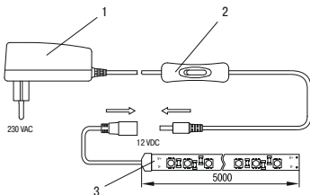
Рисунок 13 – Подключение LSR1-1-060-20-1-2XD12-S3
