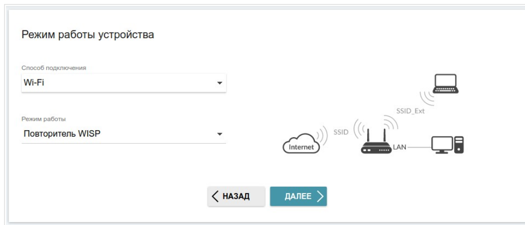
Рисунок 36. Выбор режима работы устройства. Режим Повторитель WISP .
