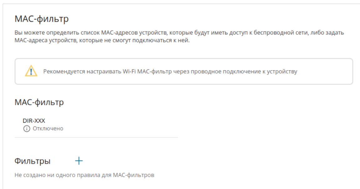
Рисунок 105. Страница для настройки MAC-фильтра для беспроводной сети.
