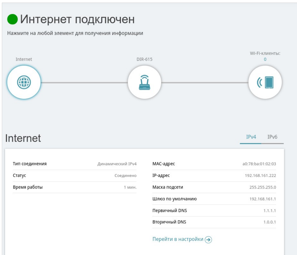
Рисунок 27. Страница Начало . Раздел Internet .
