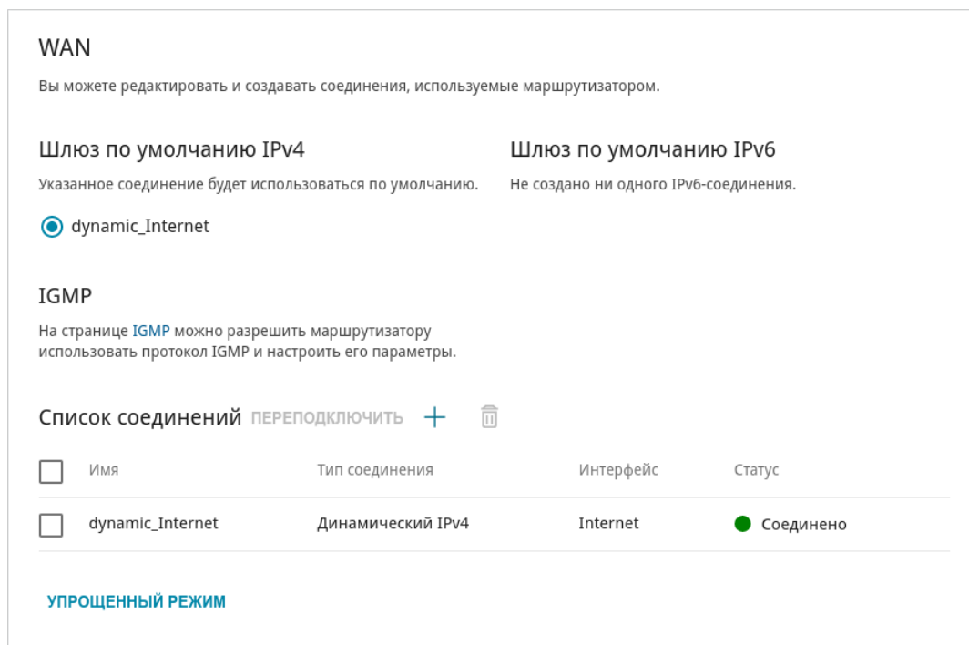
Рисунок 55. Страница Настройки / Интернет / WAN . Расширенный режим.
