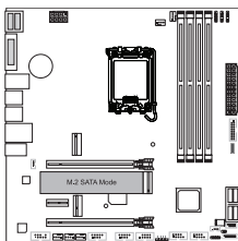
1x N/A + 1x M.2 SATA SSD Slot -- 3x SATA HDDs
