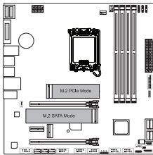
1x M.2 SATA SSD Slot + 1x M.2 PCIe SSD Slot -- 3x SATA HDDs
