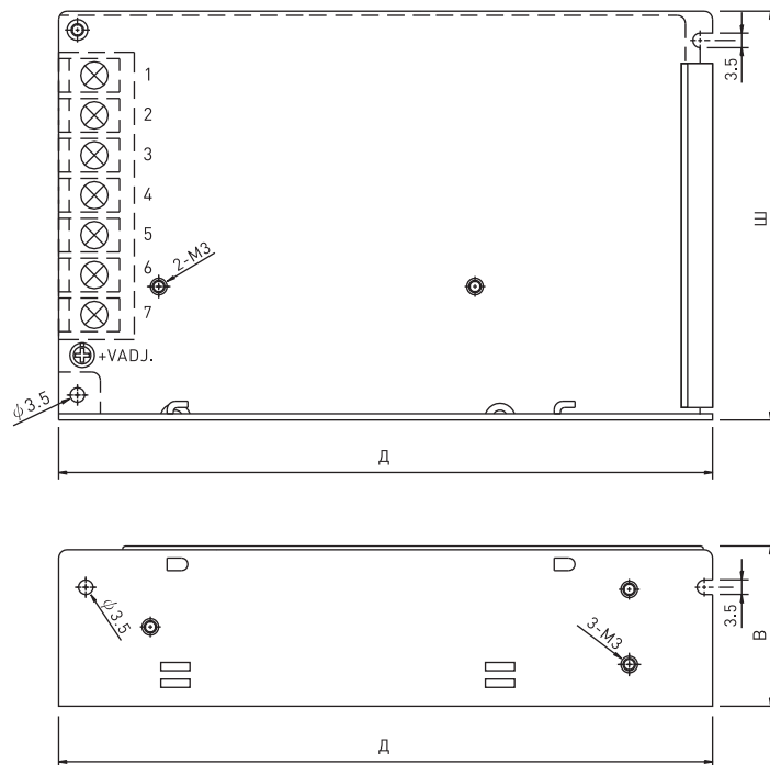
Рис.1. Габаритные размеры.
