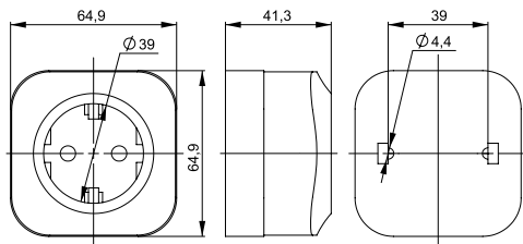
Рисунок 3 – Габаритные и установочные размеры розеток PC20-3 и РСш20-3
