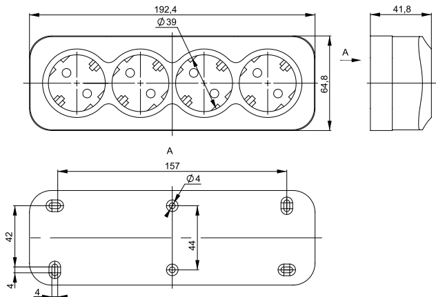
Рисунок 9 – Габаритные и установочные размеры розеток PC24-3
