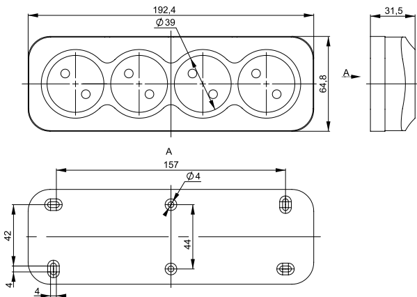
Рисунок 8 – Габаритные и установочные размеры розеток PC24-2
