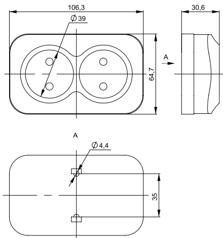
Рисунок 4 – Габаритные и установочные размеры розеток PC22-2 и РСш22-2
