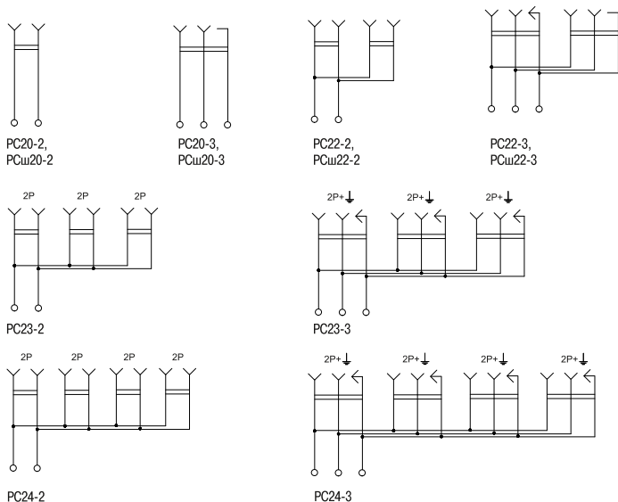
Рисунок 1 – Схемы электрические принципиальные розеток серии GLORY
