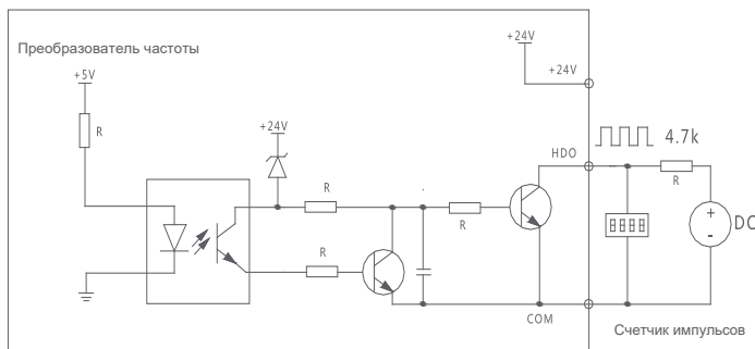
Подключение HDO через внешний источник питания
