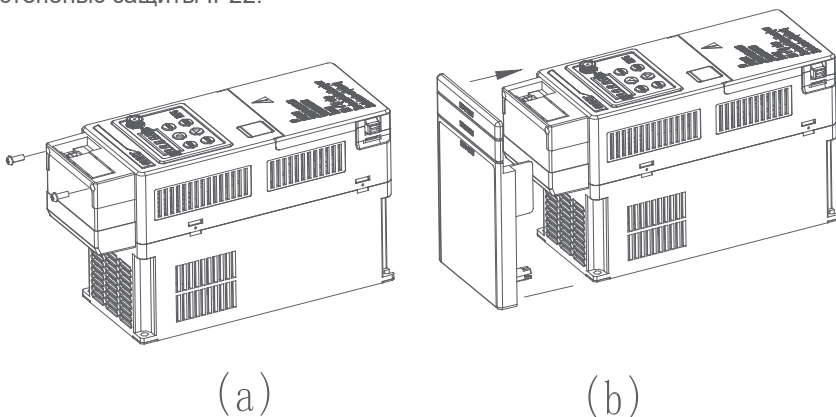
Установка кронштейна и защитной крышки.
