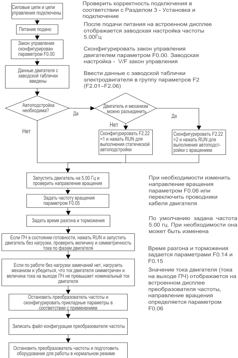
Диаграмма ускоренного запуска преобразователя частоты
