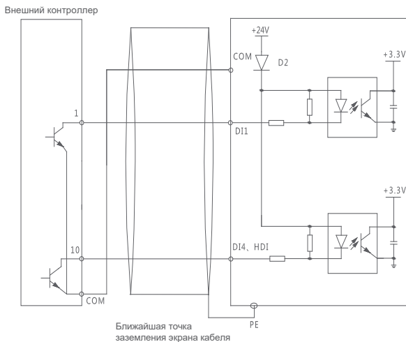
Включение дискретного входа контактом ПЛК
