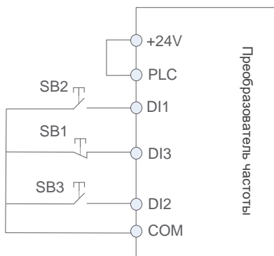
Диаграмма трехпроводного управления, режим 1
