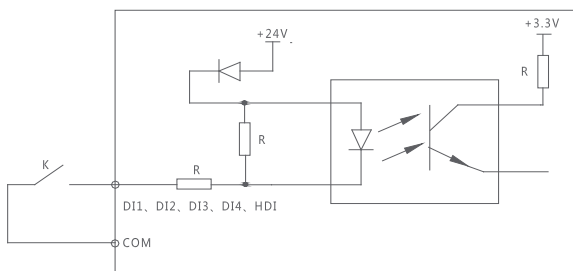
Включение дискретного входа сухим контактом
