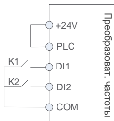
Диаграмма двухпроводного управления, режим 2
