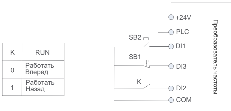
Диаграмма трехпроводного управления, режим 2
