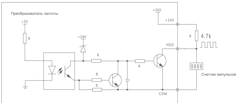
Подключение HDO через внутренний источник питания
