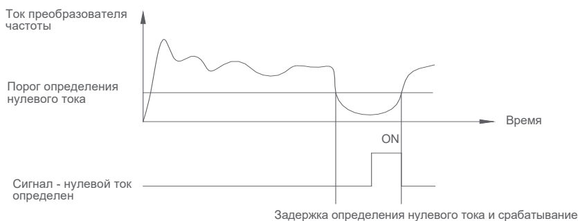
Диаграмма определения нулевого тока двигателя
