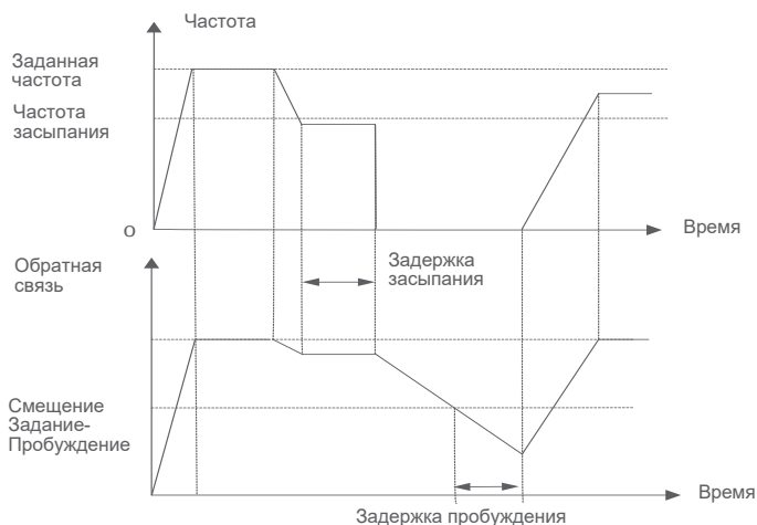
Диаграмма работы спящего режима
