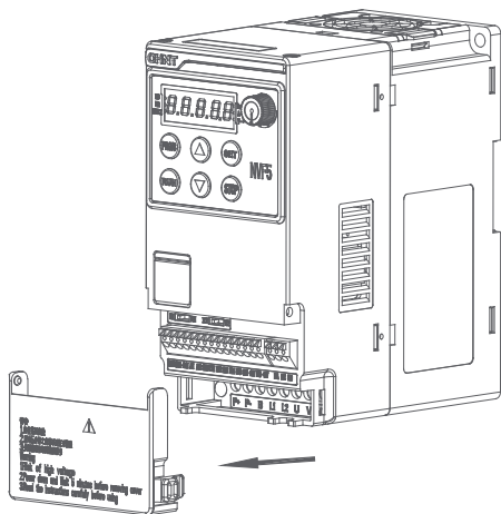
Крышка клеммника NVF5-0.4/TD2 ~ NVF5-2.2/TS4-B
