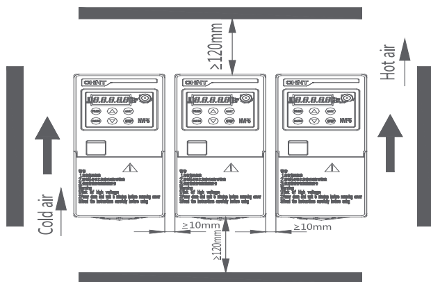
Минимальные расстояния при установке вплотную
