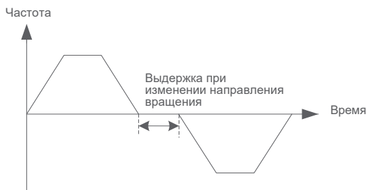
Диаграмма задержки переключения направления вращения
