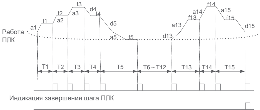
Диаграмма работы ПЛК как источника задания частоты
