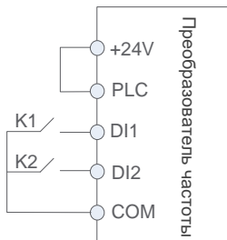
Диаграмма двухпроводного управления, режим 1
