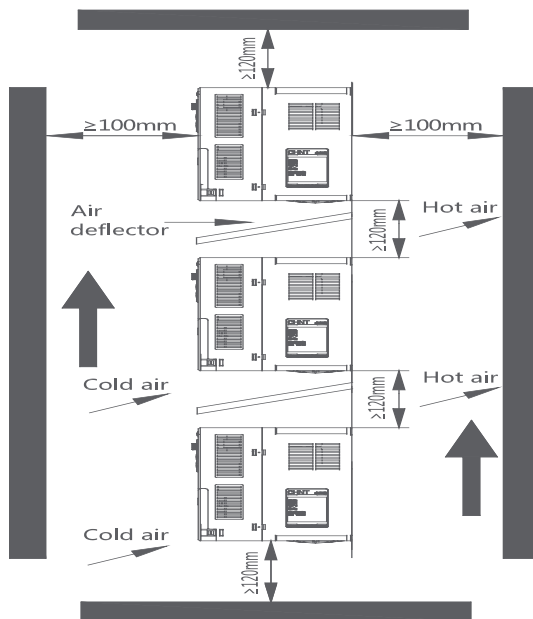
Минимальные расстояния при вертикальном монтаже
