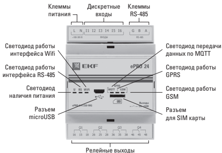
Рисунок 1. Внешний вид контроллера ePRO-6-4-230-W
