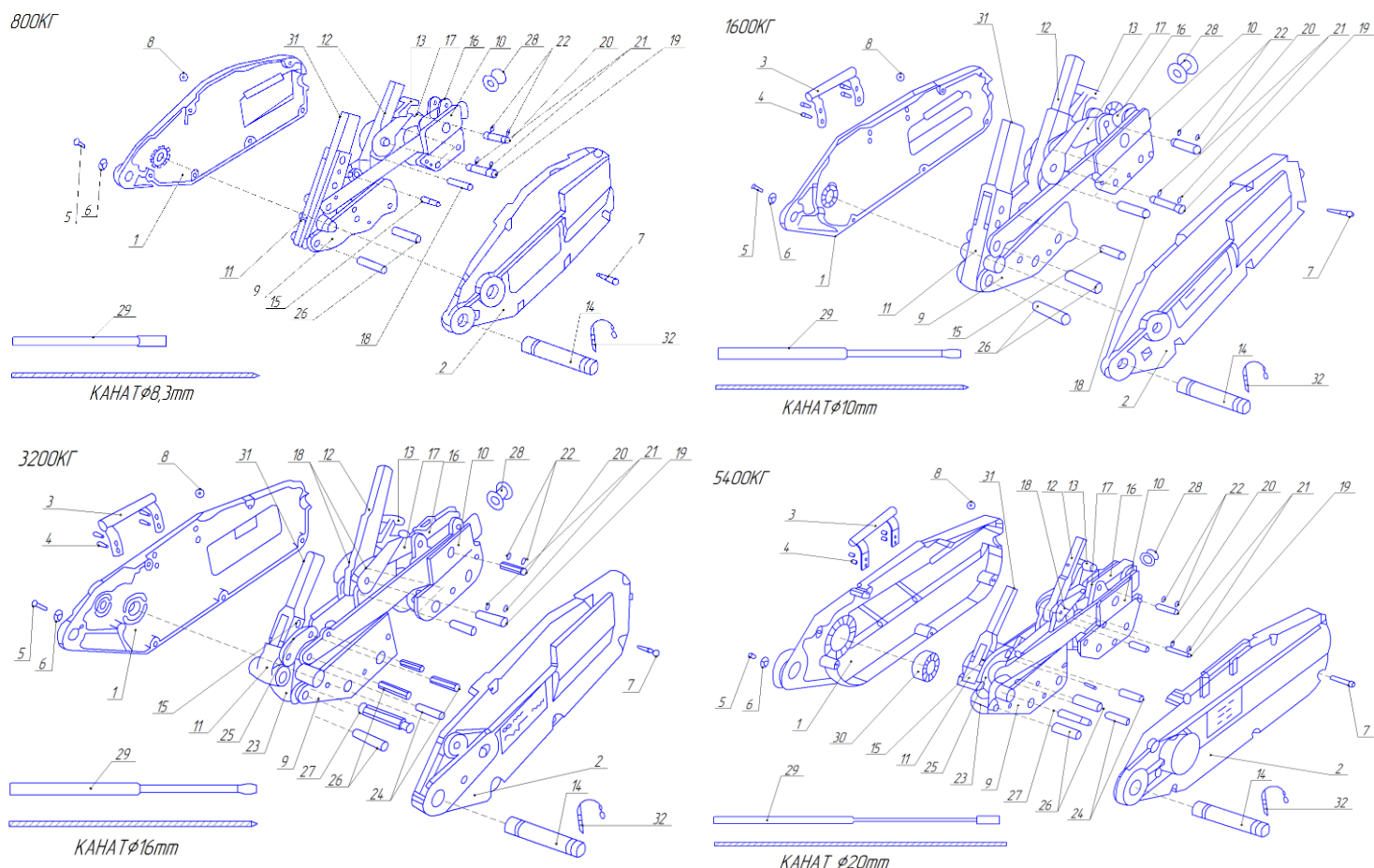
Рисунок 2. Взрыв схемы МТМ 0,8 – 5,4 т.
