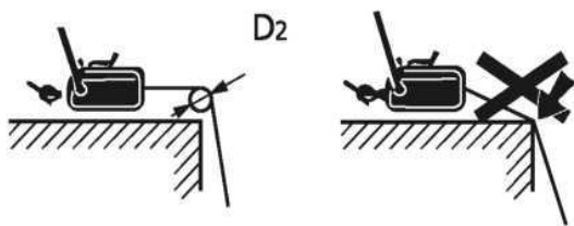
Рисунок 3. Подтягивание груза при помощи МТМ.
