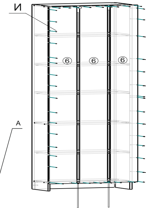
Схема установки соединителя задней стенки
