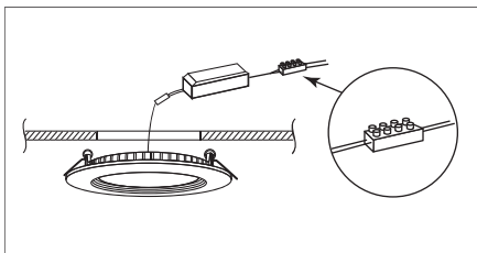
5. Подключите светильник с драйвером к электрической сети и установите в подготовленное отверстие.
