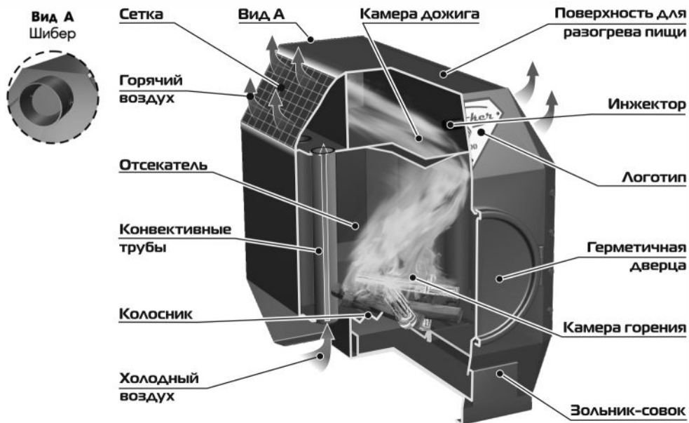
Рисунок - 1. Схема работы печей длительного горения.
