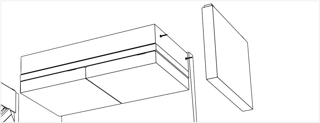
1. Соединить подлокотники с помощью 4-х болтов М8х60.
