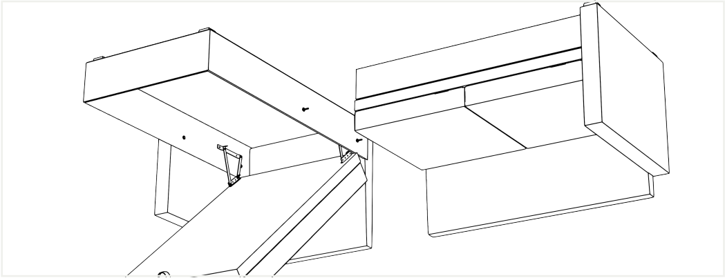
2. Соединить основную часть с оттоманкой 2-мя болтами М8х35.
