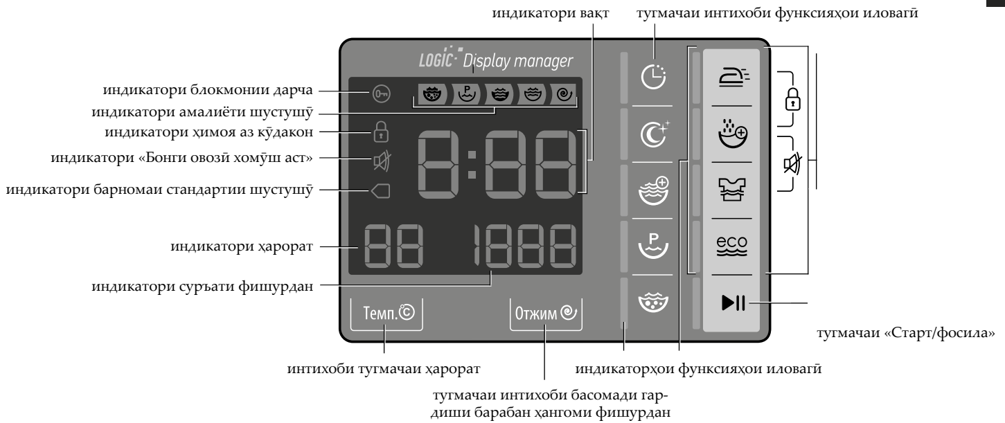
Расми 3 – Ҳудуди индикаторҳо ва тугмаҳои идоракунии
