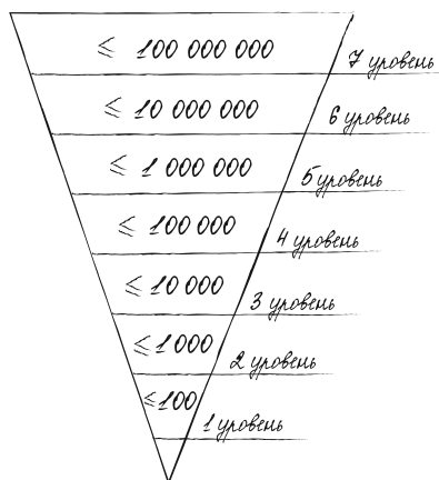
Рис. 1. Уровни мужской энергии
