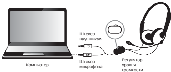
Рис. 1. Схема подключения
