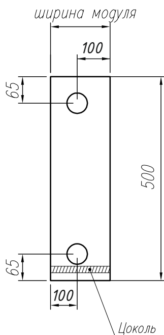
Рис.5 Схема установки опор
