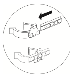
Рис.9 Схема монтажа клипс на цоколь
