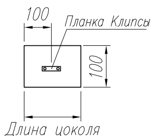
Рис.9 Схема монтажа клипс на цоколь
