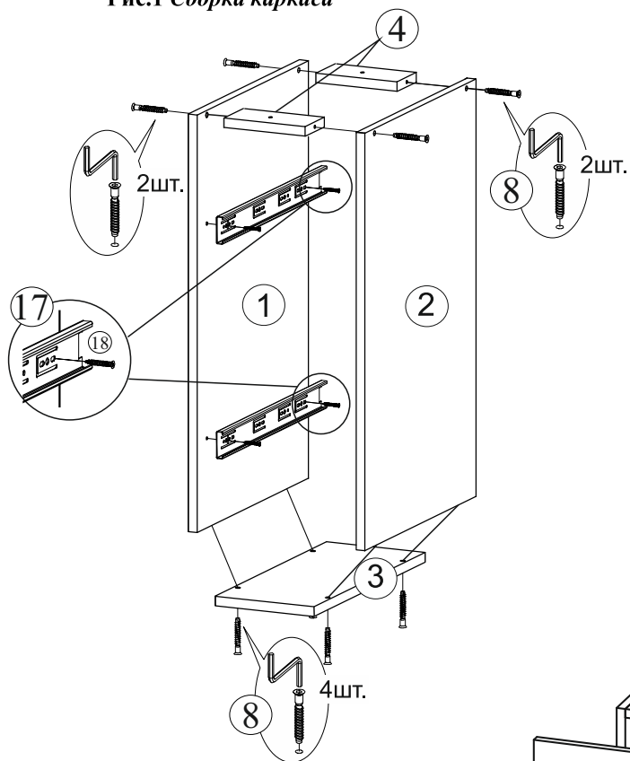
Рис.1 Сборка каркаса
