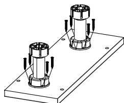
Рис.5 Схема установки опор
