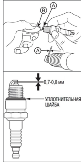
Рис. 23 Зазор между электродами свечи зажигания
