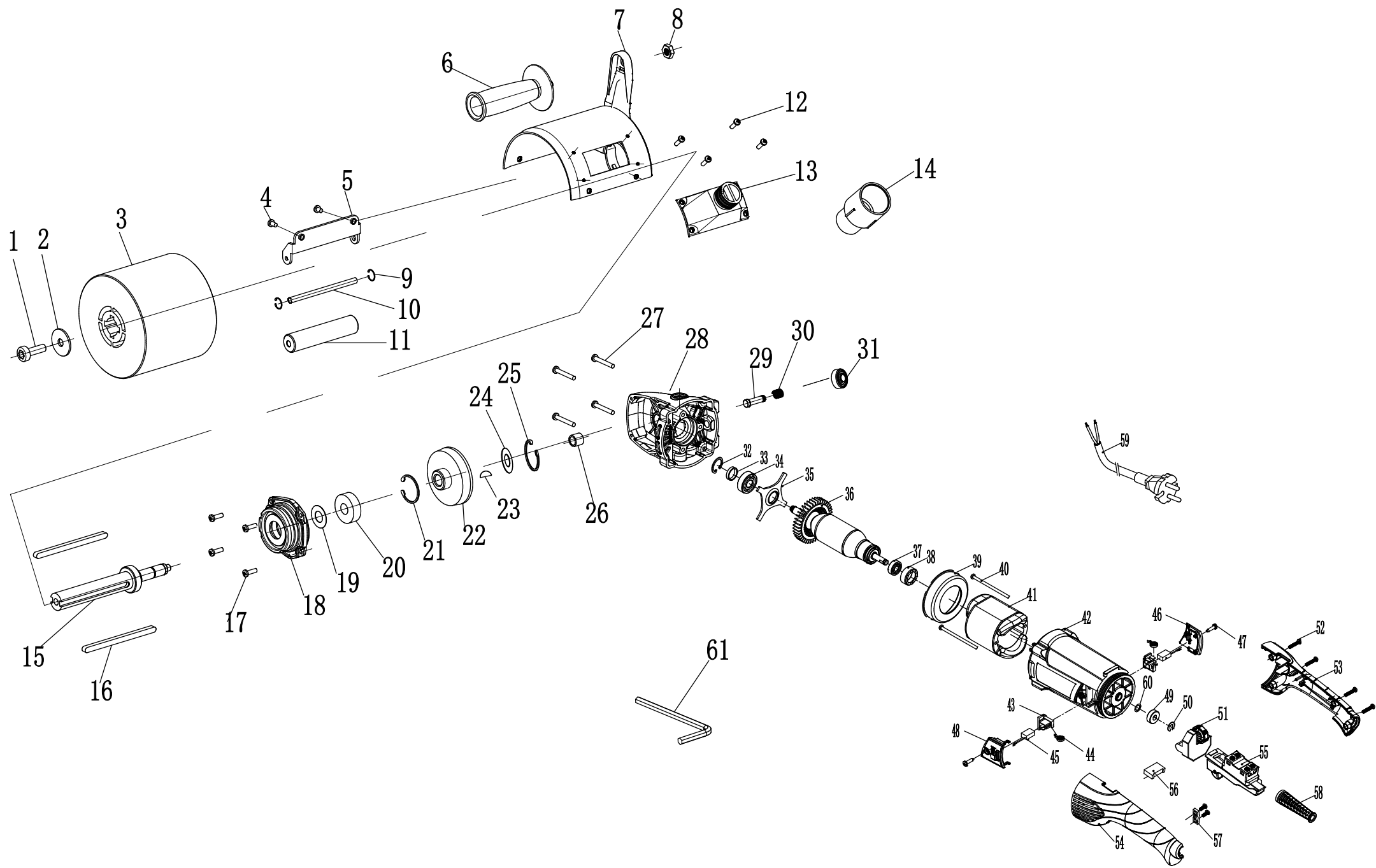
WT8821拉丝机爆炸图-FELISATTI专用 版本:00
