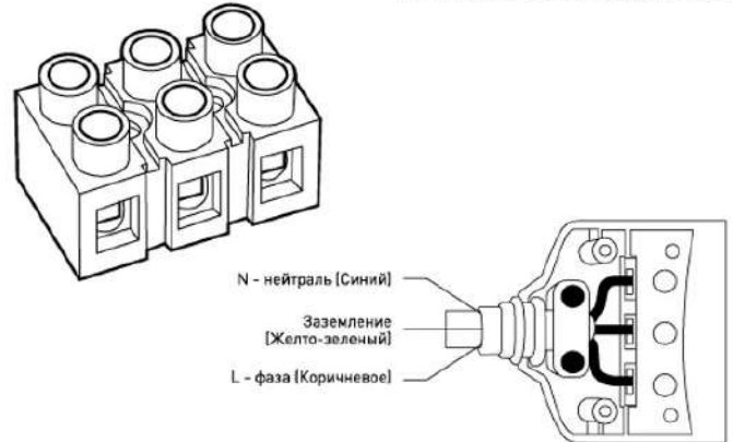
Рис.1. Подключение сетевого провода к колодке.
