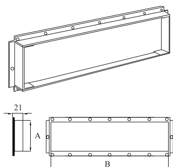
Рис. 9. Приточный фланец
