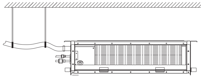
Неправильный монтаж
