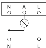
Рисунок 5 – Схема подключения датчика ДД 025, ДД 027
