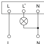
Рисунок 9 – Схема подключения датчика ДД 401
