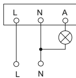
Рисунок 7 – Схема подключения датчика ДД 201
