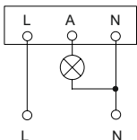
Рисунок 8 – Схема подключения датчика ДД 301
