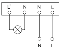
Рисунок 6 – Схема подключения датчика ДД 026
