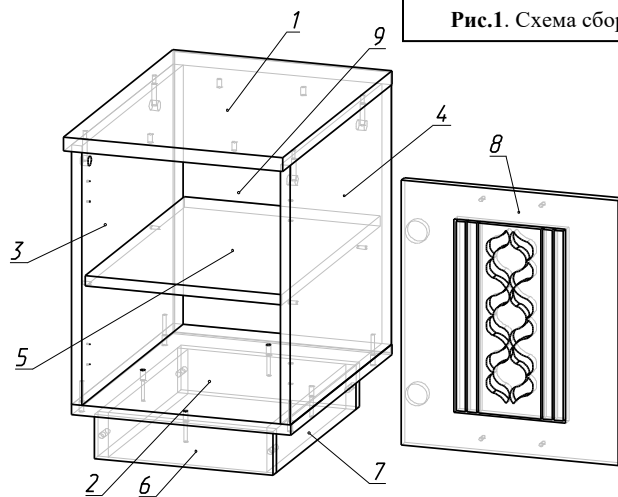
Рис.1. Схема сборки
