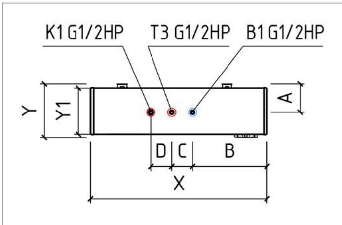
Вид сверху с прорисовкой нижних выпусков
