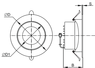
Рисунок 1 – Габаритные размеры ДВО 1811 PRO – ДВО 1813 PRO
