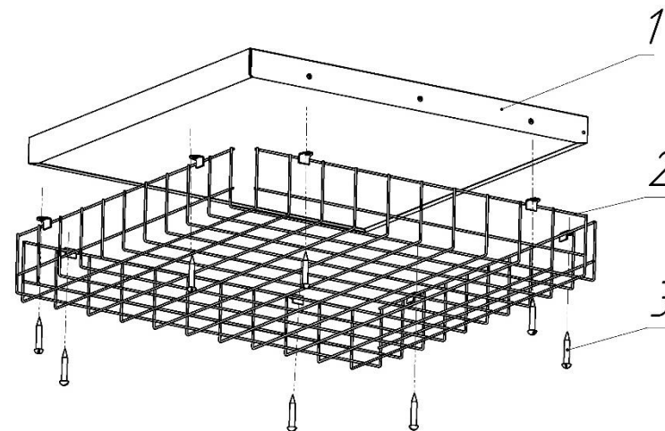
Рисунок 1. Схема монтажа защитной решётки
