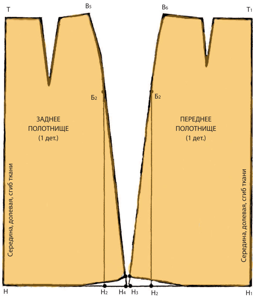
Выкройка расклешенной юбки
