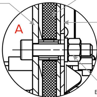
Панель термоизоляционная
