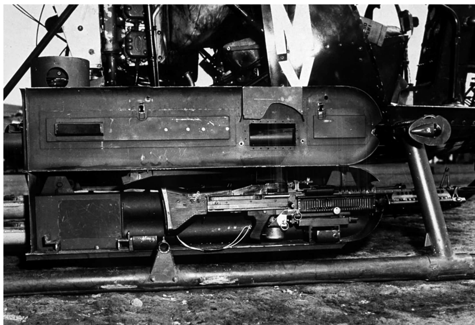
Ракетно-пулеметный контейнер, подвешенный на вертолете Н-13.
