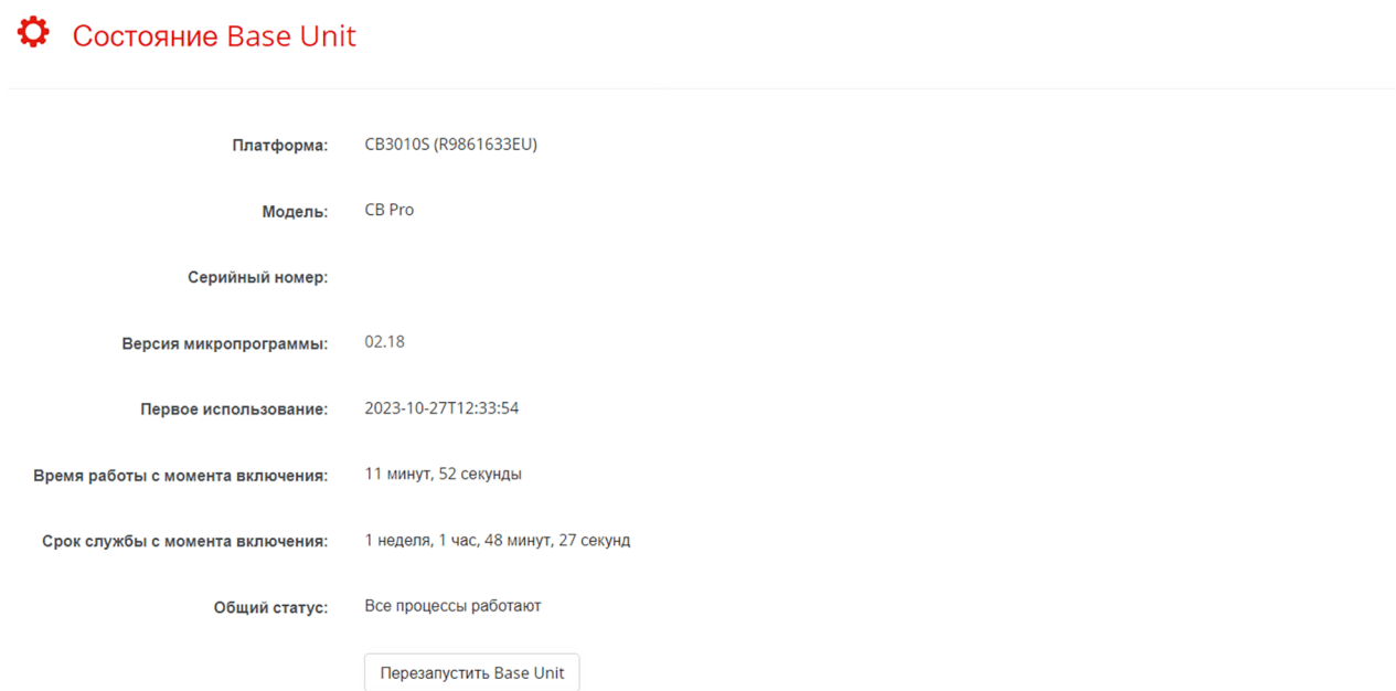
Изображение 6–45 Пример состояния Base Unit
