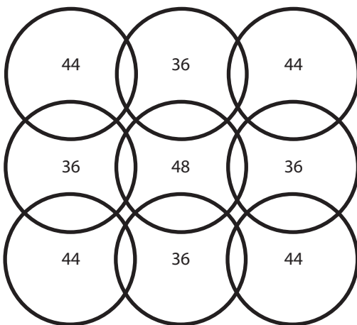
Изображение 6–30 Пример перекрытия каналов на частоте 5 ГГц
