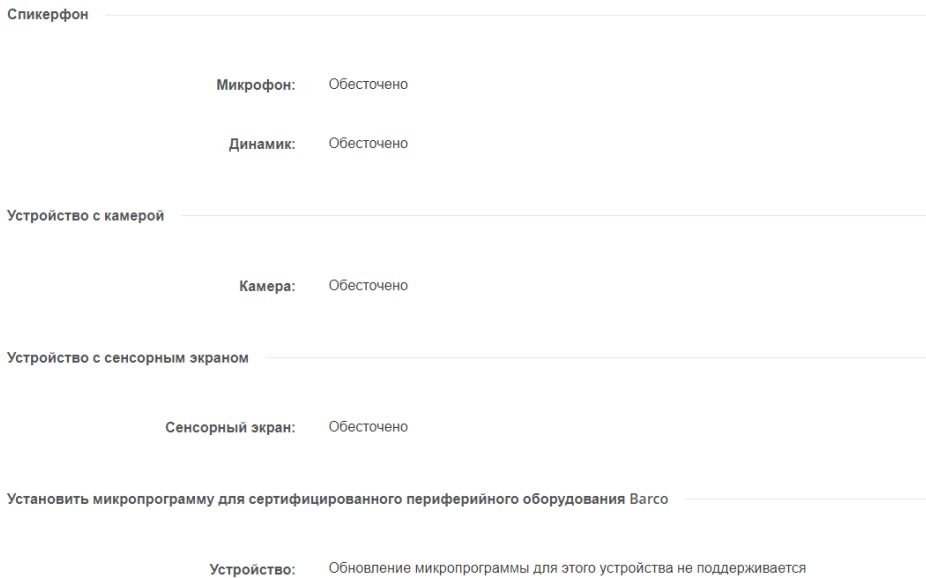
Изображение 6–22 Пример страницы периферийных устройств
