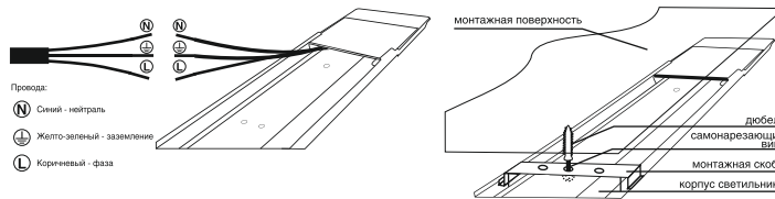
Рисунок 1 Подключение к сети
