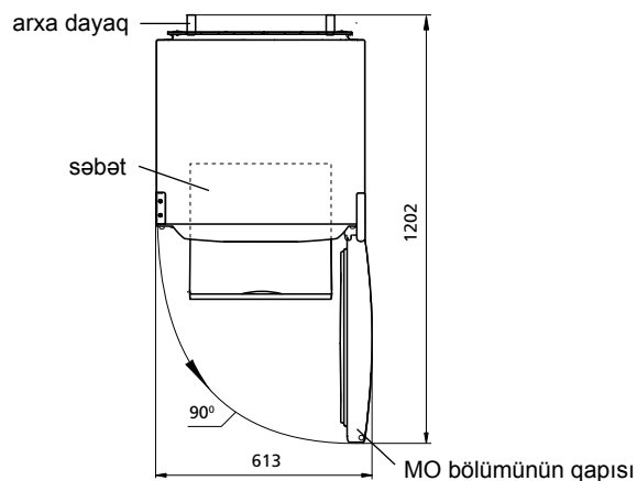
Rəsim 2 – Soyuducu (üstəndən görünüşü)
