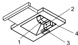
Рис. 2а. Kamilla slim 500, Kamilla slim 600, Slim60ix MB
