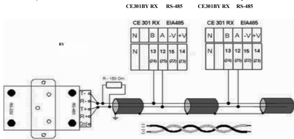
Рисунок 3.4 – Схема подключения счетчика CE301BY RX с интерфейсом RS-485 через внешний адаптер RS-485/RS-232 к COM-порту ПЭВМ
