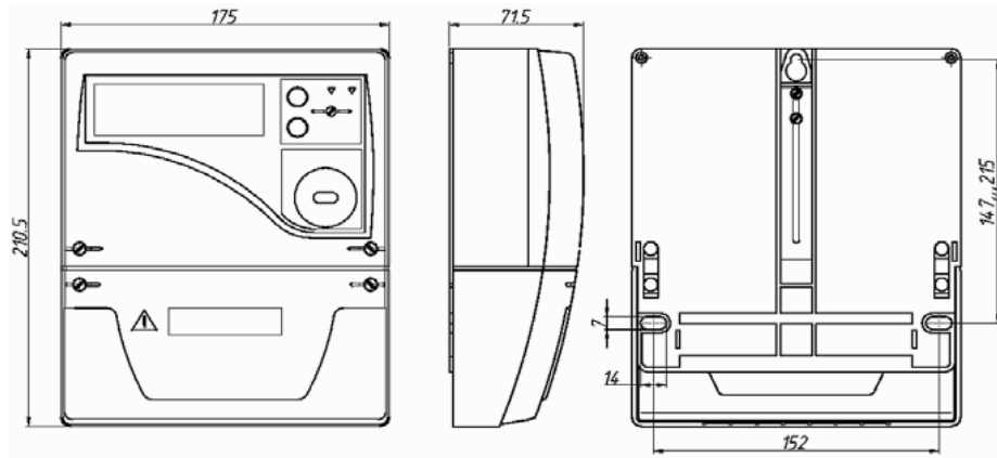
Общий вид счетчика исполнения СЕ301ВУ S31
