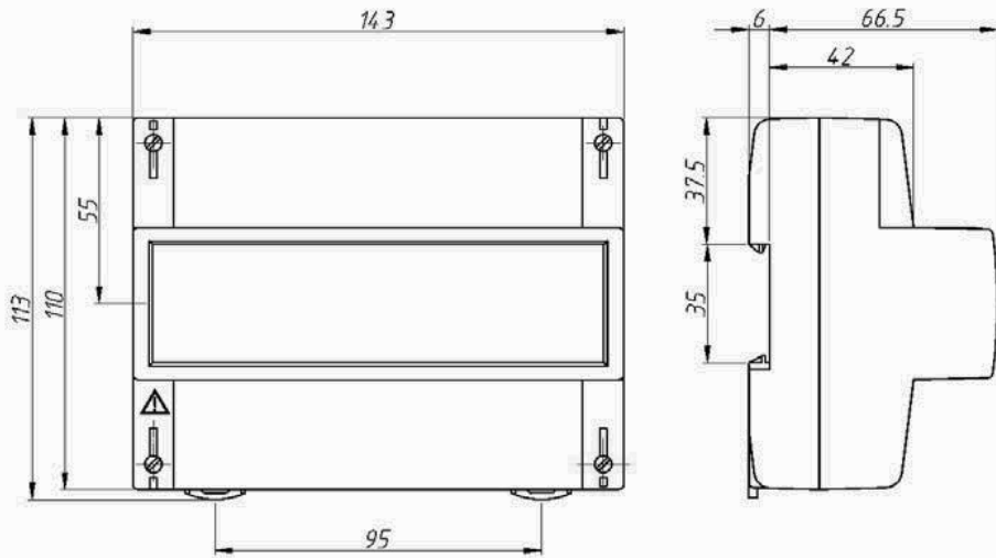
Общий вид счетчика исполнения СЕ301ВУ R31
